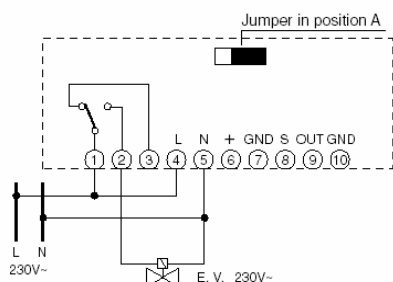
Koblingskjema med manuel reset magnetventil normalt åpen. 230VAC (Ref. 1450/500).
