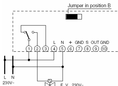
Koblingskjema med manuel reset magnetventil normalt lukket. 230VAC
